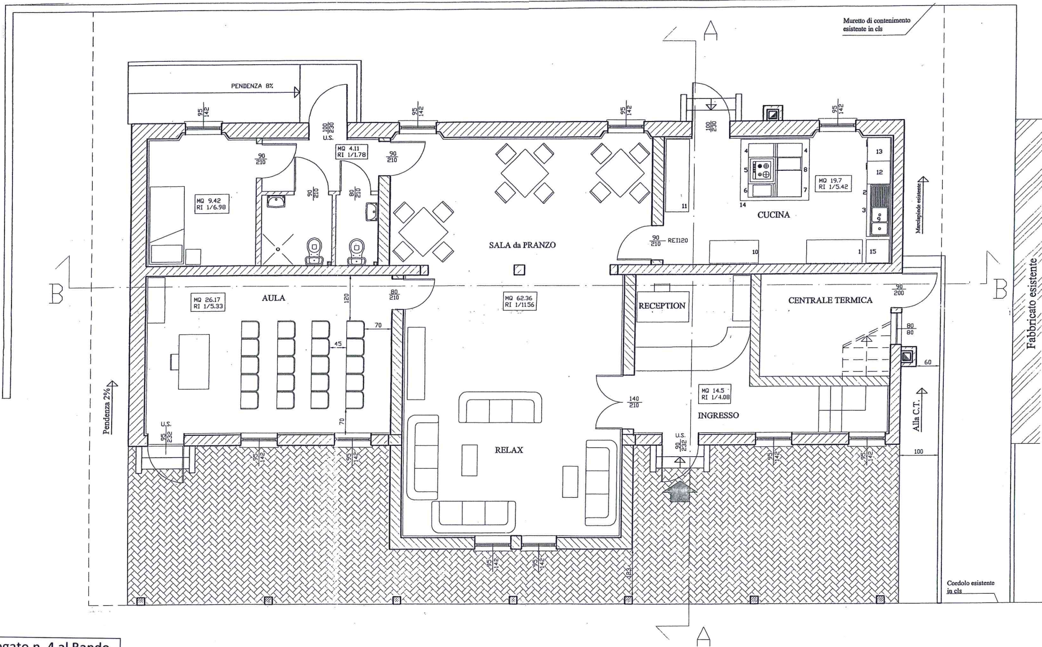
Allegato n. 4 al Bando Casa per Ferie Fontane pianta piano terra foglio A4, scala 1:100
